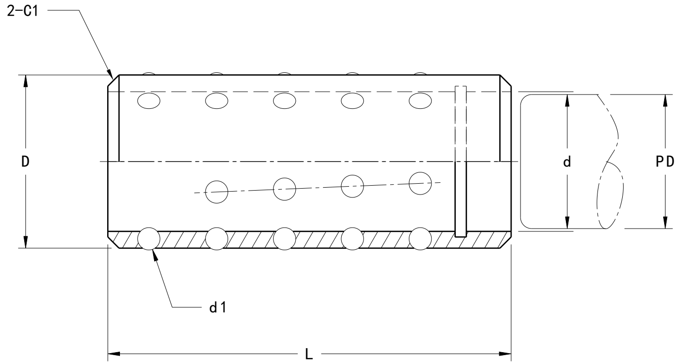
Section view A-A Scale: 3:1
