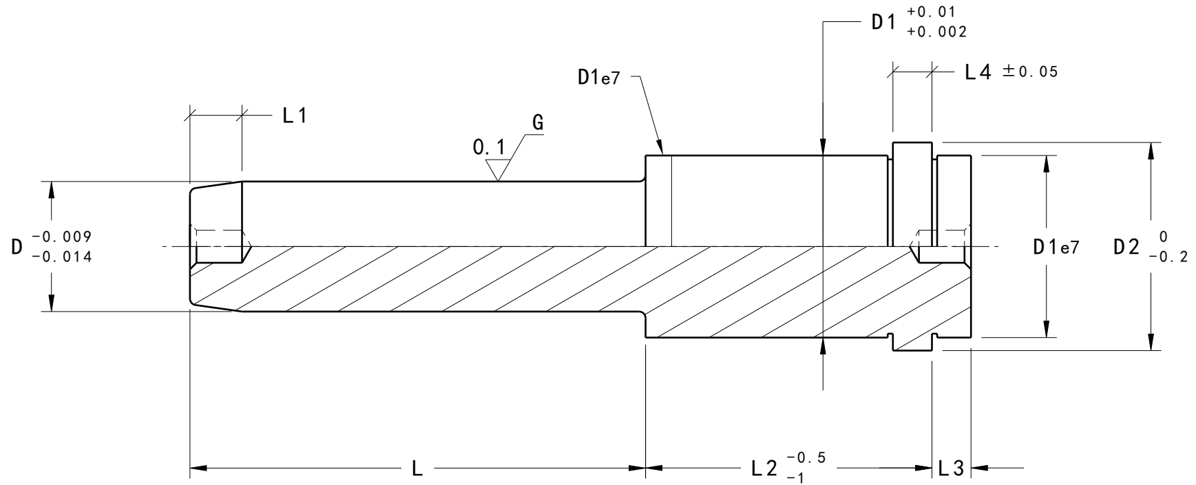
剖面視圖A-A 縮放: 5:2
