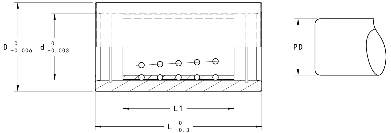
Section view A-A Scale: 3:1
