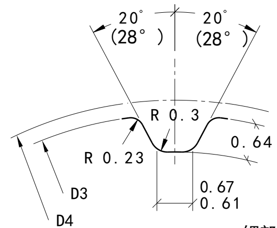
細部 B 縮放: 15:1
