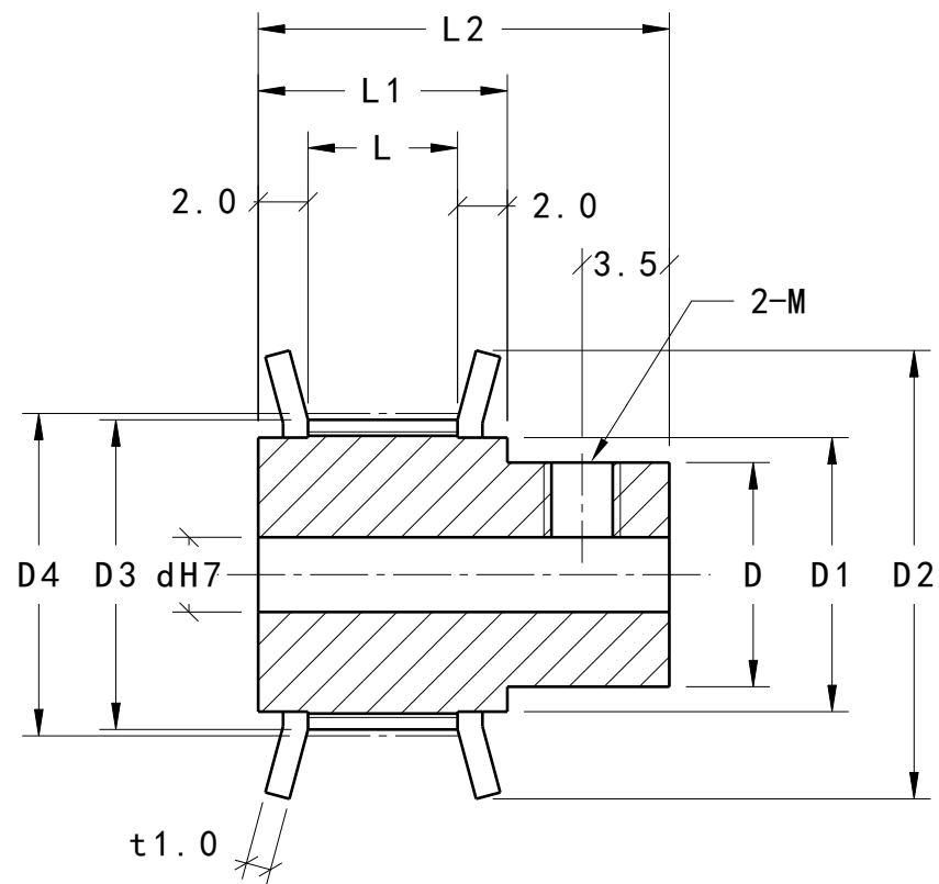
剖面視圖A-A 縮放: 3:1
