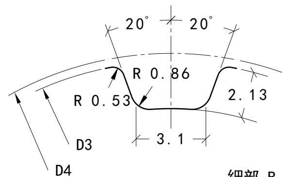
細部 B 縮放: 6:1
