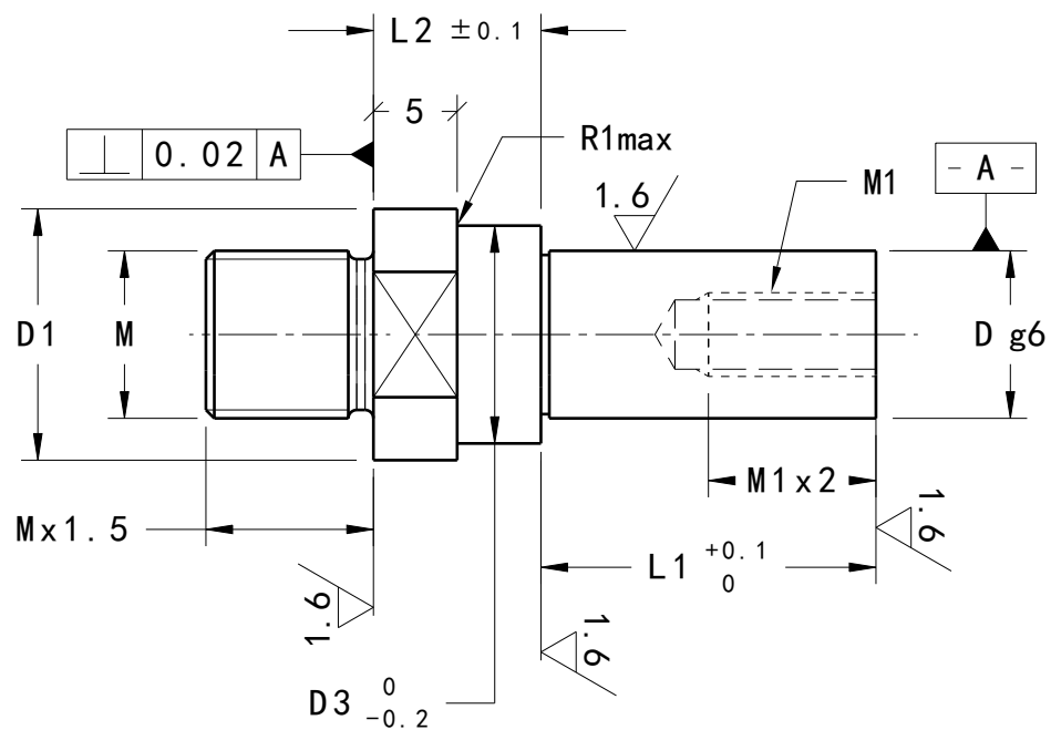
Right view Scale: 2:1
