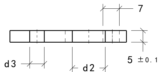
剖面視圖B-B 縮放: 1:1
