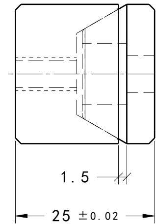
前視圖 縮放: 3:2
