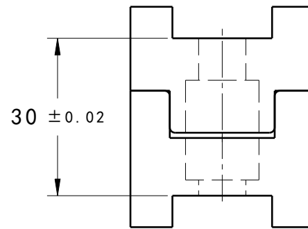
前視圖 縮放: 1:1
