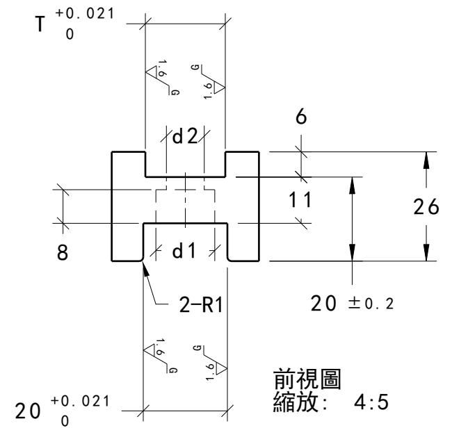
前視圖 縮放: 4:5
