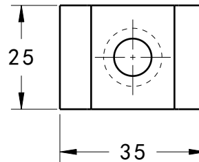
前視圖 縮放: 4:5
