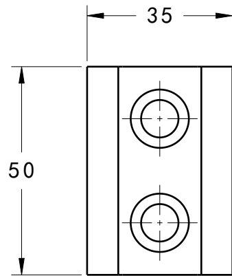
前視圖 縮放: 4:5
