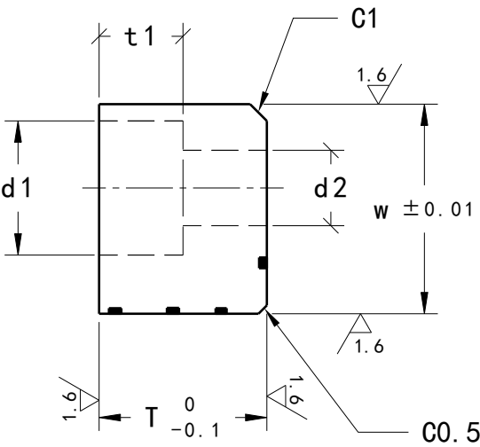
前視圖 縮放: 5:2
