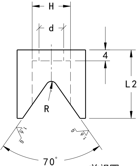
前視圖 縮放: 6:5
