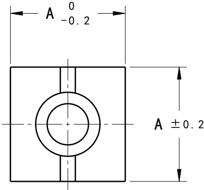
前視圖 縮放: 6:5
