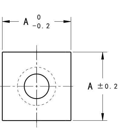
前視圖 縮放: 6:5
