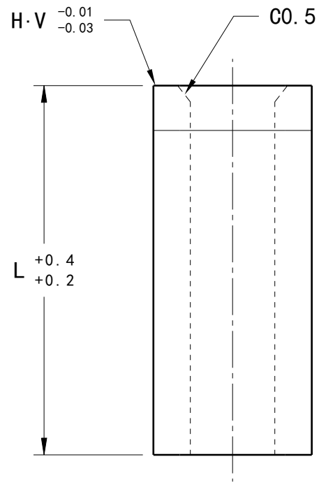
前視圖 縮放: 10:1
