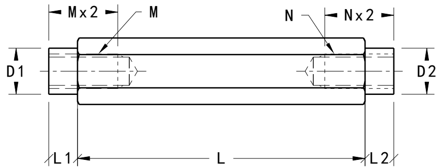
前視圖 縮放: 3:2
