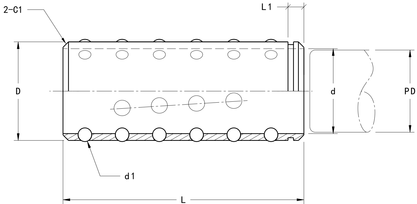
Section view A-A Scale: 5:2
